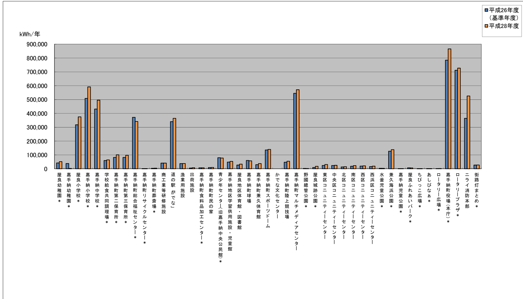
図 1-4 施設別電気使用量と経年変化(900,000kWh/年以下) (平成26年度、平成28年)
