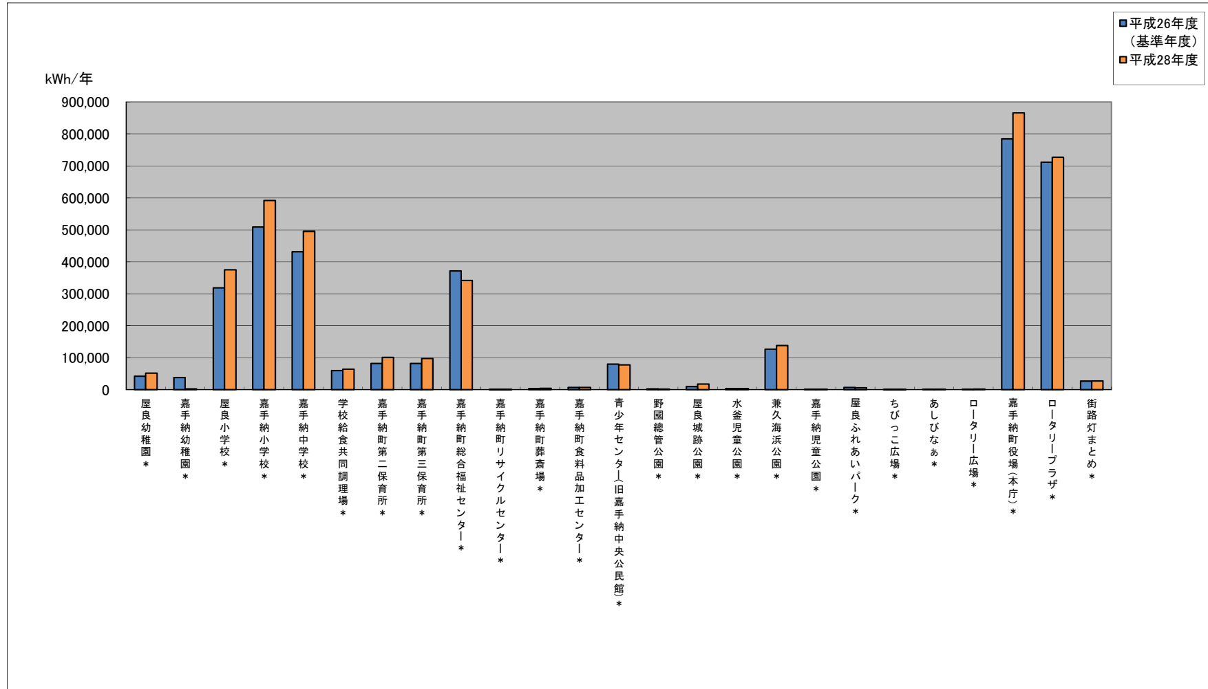
図1-5 対象施設別電気使用量と経年変化（平成26年度、平成28年）
