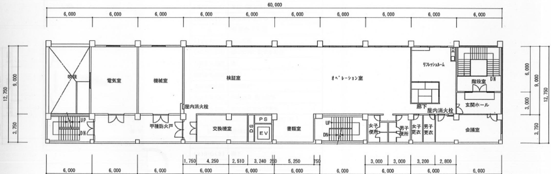
2階平面図 S=1:250
