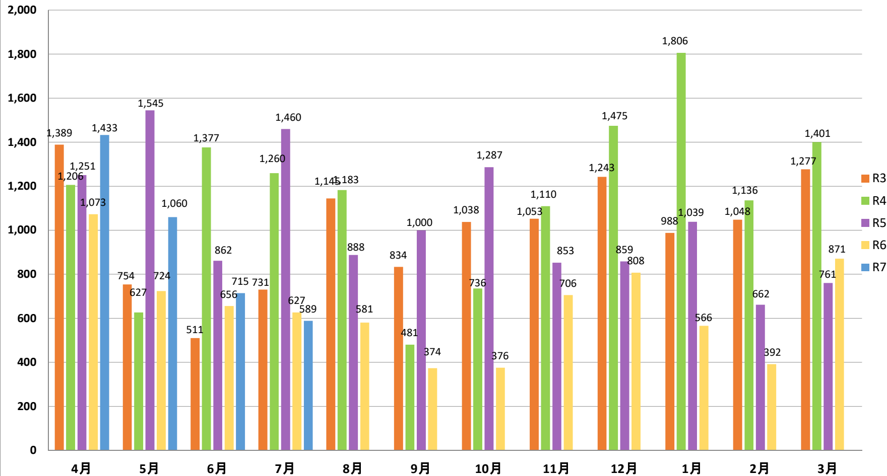
騒音発生回数(屋良局)
